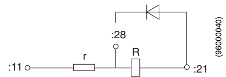
Fig. 2 RXMS 1
